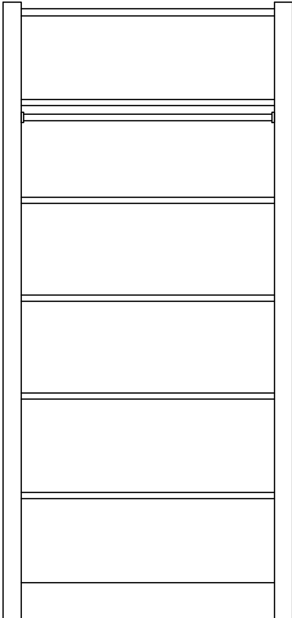
Kétajtós szekrény, 4 db polccal, 1 db vállfatartó rúddal
