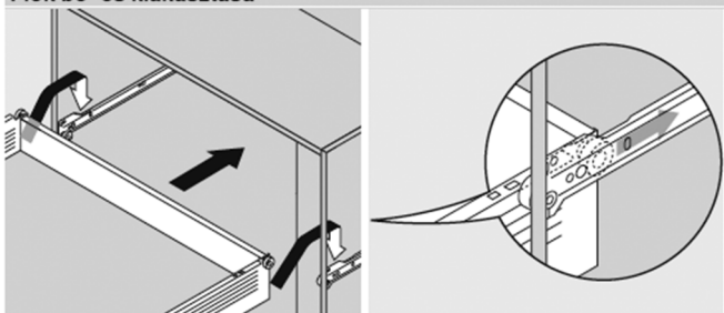
Fiók be- és kiakasztása
